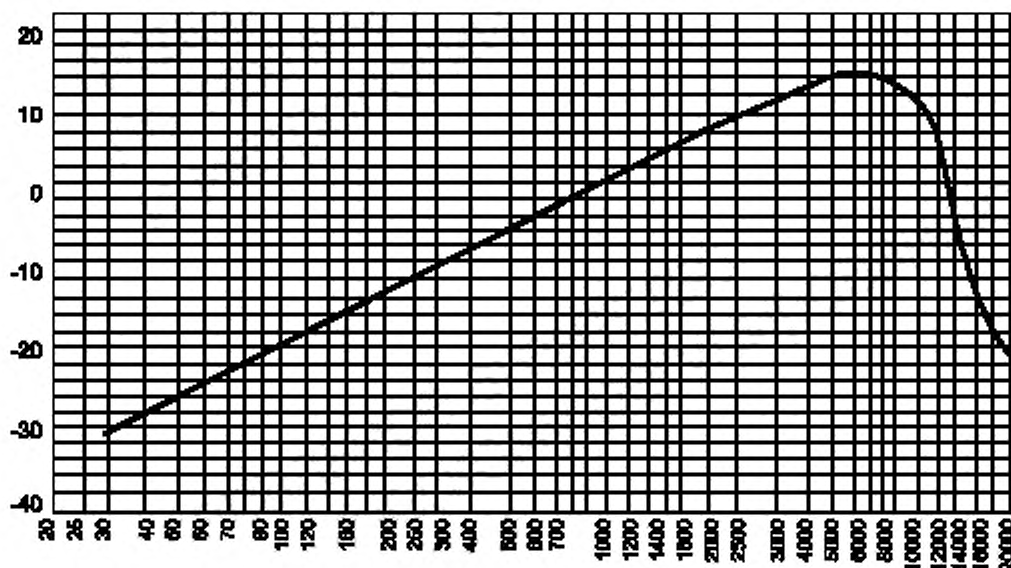
Рисунок 19 — График АЧХ псофометрического фильтра в соответствии с [1]
