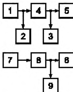
1 — низкочастотный генератор сигналов; 2, 3 — вольтметры; 4 — тракт, вносящий помеху; 5, 6 — номинальные сопротивления нагрузки — резистор; 7 — резистор — эквивалент сопротивления источника; 8 — испытываемый тракт; 9 — анализатор спектра или селективный вольтметр
