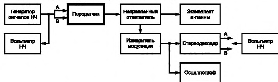
Рисунок 29 — Схема измерения неравномерности АЧХ в режиме СТЕРЕО
