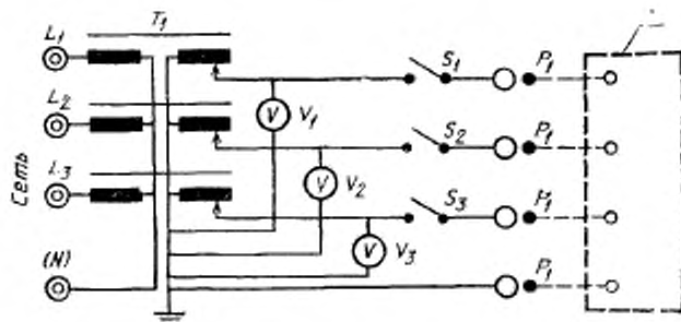
Измерительная цепь питания для многофазного ИЗДЕЛИЯ, предназначенного для соединения с многофазной ПИТАЮЩЕЙ СЕТЬЮ (см. п. 19.4б)
