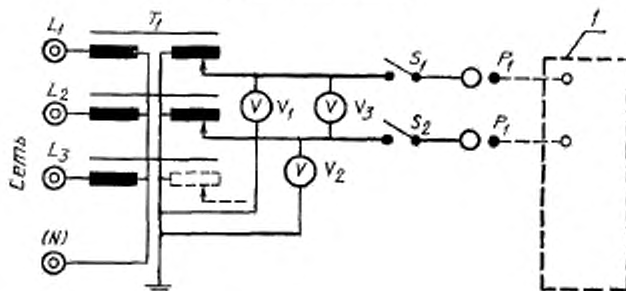
Измерительная цепь питания для однофазного ИЗДЕЛИЯ, предназначенного для соединения с многофазной ПИТАЮЩЕЙ СЕТЬЮ (см. п. 19.4б)
