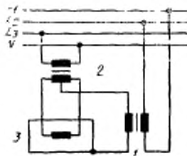
1 — испытательный трансформатор; 2 — разделительный трансформатор; 3 — ИЗДЕЛИЕ
