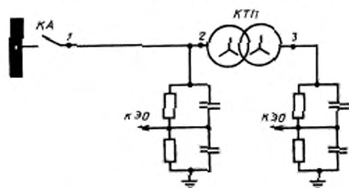
Схема коммутации высокого напряжения
