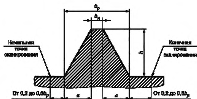
b_н — ширина нижнего основания выступа; b_в — ширина верхнего основания выступа; h — высота выступа, a — значение проекции наклонной стенки на плоскость нижнего основания выступа
