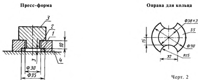
1 — кольцо; 2 — форма; 3 — пуансон, 4 — калка
