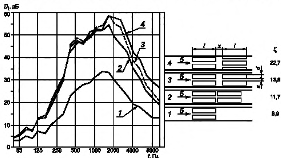
l = 0,75 м; s = 0,1 м; 1 — 4 — варианты расположения пластин; x = 0,1 м; d = 0,2 м; 5 — направление потока
