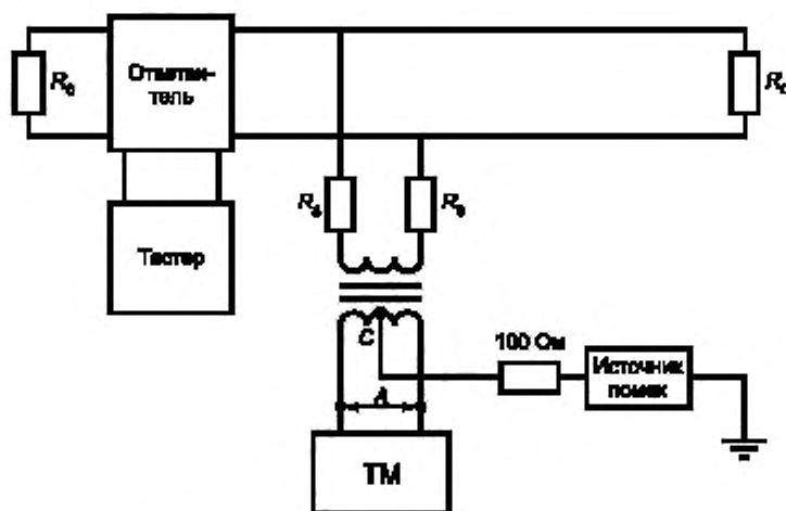
Рисунок 5 — Схема тестирования входного сигнала при синфазных помехах и трансформаторном подключении ТМ
