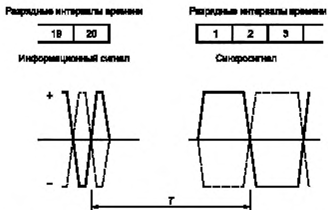
Рисунок 7 — Измерение временных пауз при передаче информации
