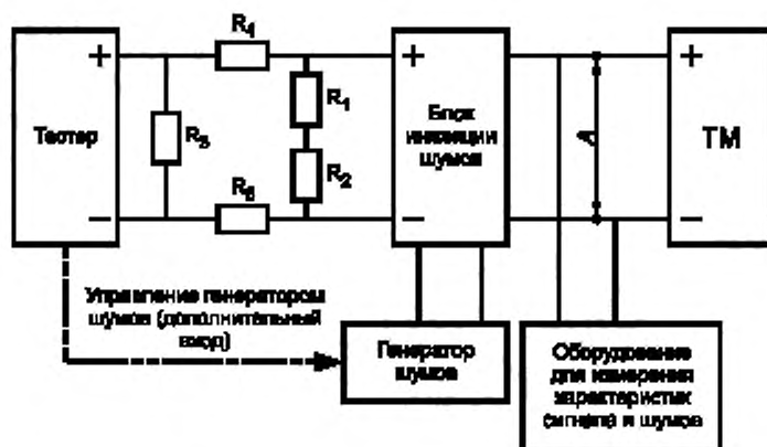
Рисунок 8 — Схема тестирования помехоустойчивости ТМ
