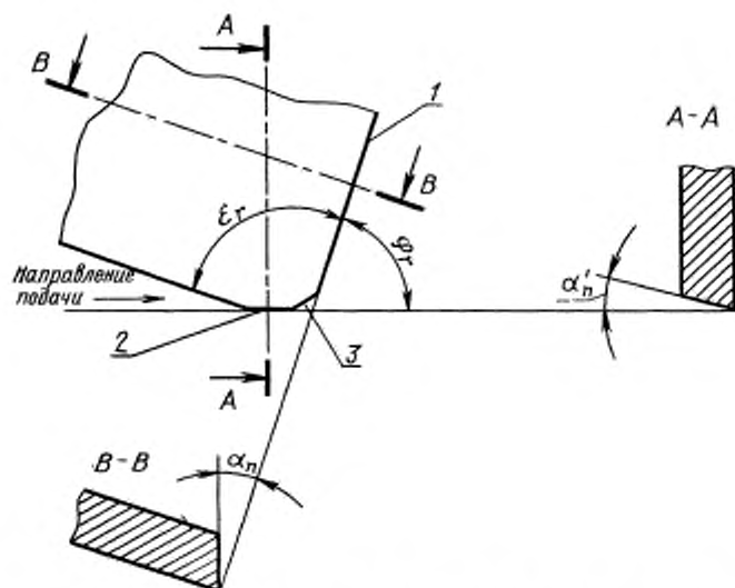
Т — главная режущая кромка; 2 — зачистная режущая фаска; 3 — переходная фаска Черт. 4
