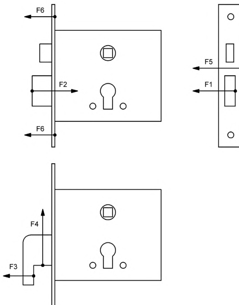
Рисунок 1 — Точки приложения сил, воздействующих на механизм замка
