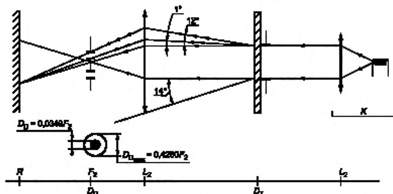
Рисунок 1 — Схема измерения коэффициента рассеивания и пропускания света
