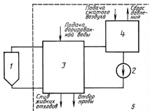
1 — пенал; 2 — насос; 3 — система управления; 4 — компенсатор давления; 5 — арматурный блок
