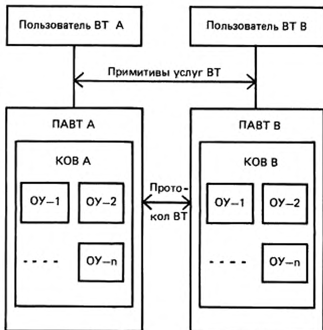
Рисунок 2 — Объекты управления в модели протокола ВТ
