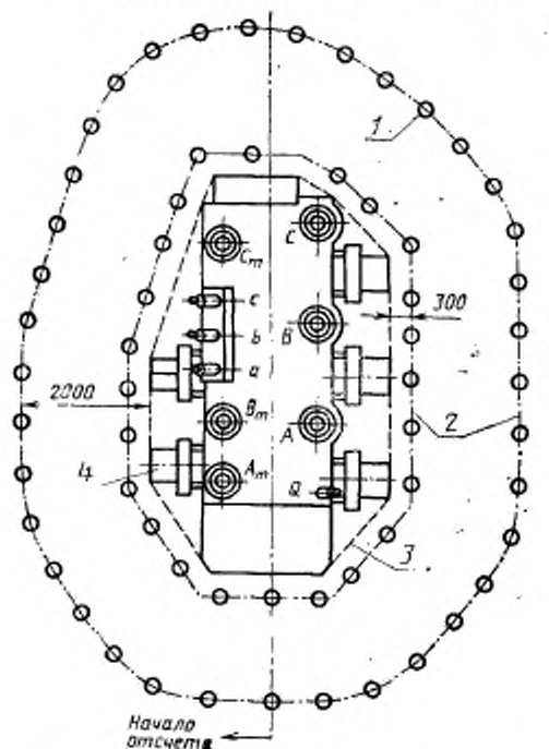
1 — микрофон; 2 — измерительная линия; 3 — излучающая поверхность; 4 — охладитель
