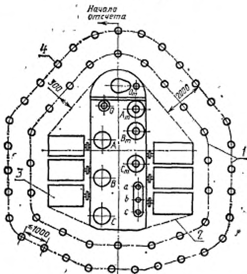
1 — измерительная линия; 2 — излучающая поверхность; 3 — охладители; 4 — микрофон
