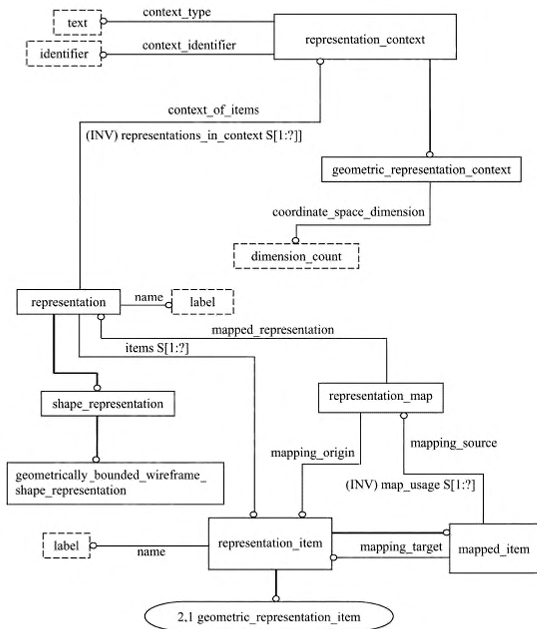
Рисунок С.1 — alc_geometrically_bounded_wireframe — EXPRESS-G диаграмма 1 из 6
