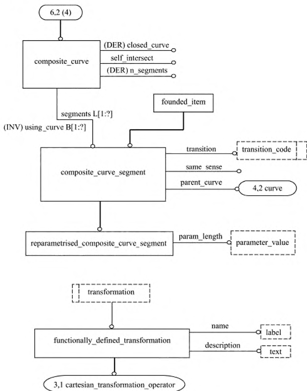
Рисунок С.6 — alic_geometrically_bounded_wireframe — EXPRESS-G диаграмма 6 из 6
