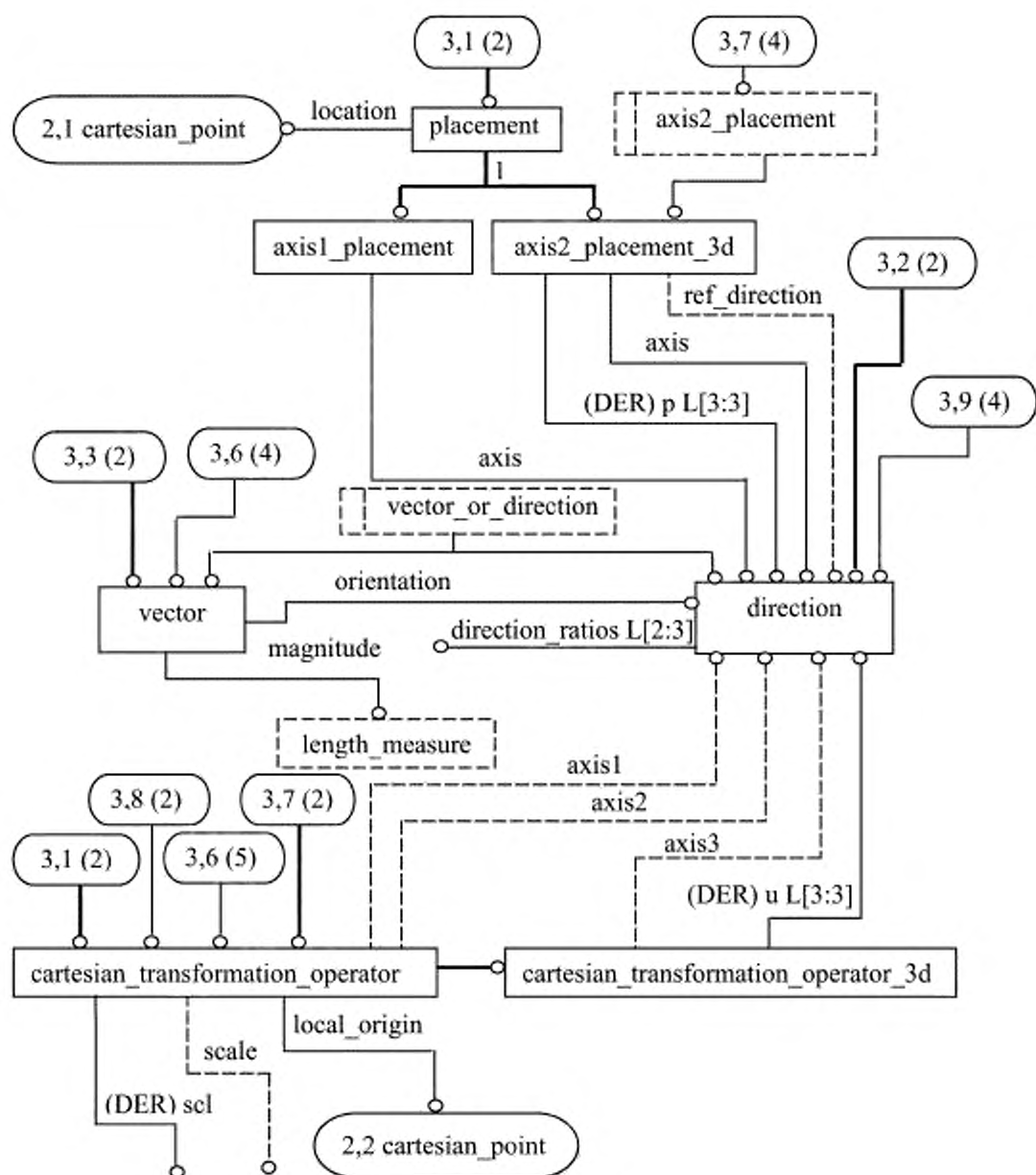
Рисунок С.3 — alc_geometrically_bounded_wireframe — EXPRESS-G диаграмма 3 из 6
