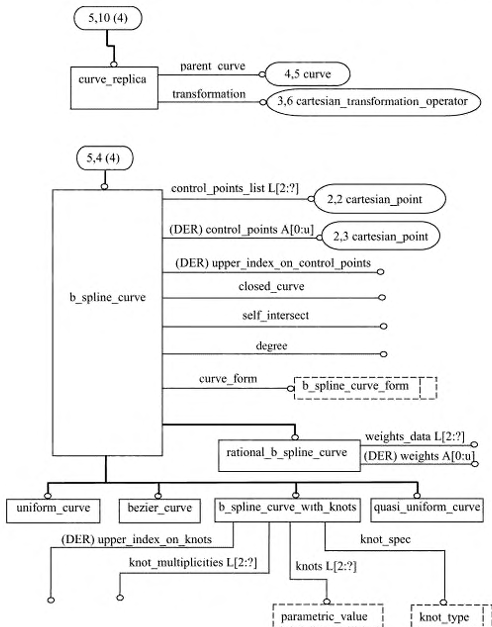
Рисунок С.5 — alic_geometrically_bounded_wireframe — EXPRESS-G диаграмма 5 из 6
