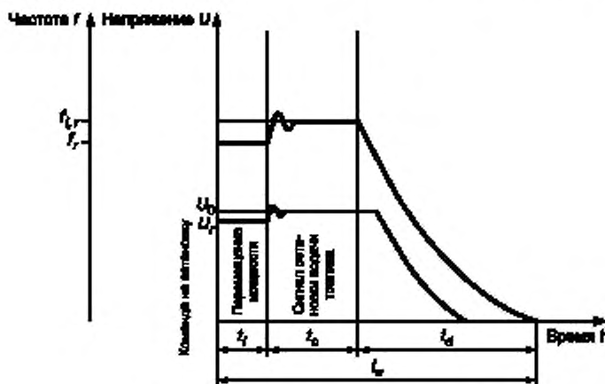
Рисунок 11 — Характеристики остановки
