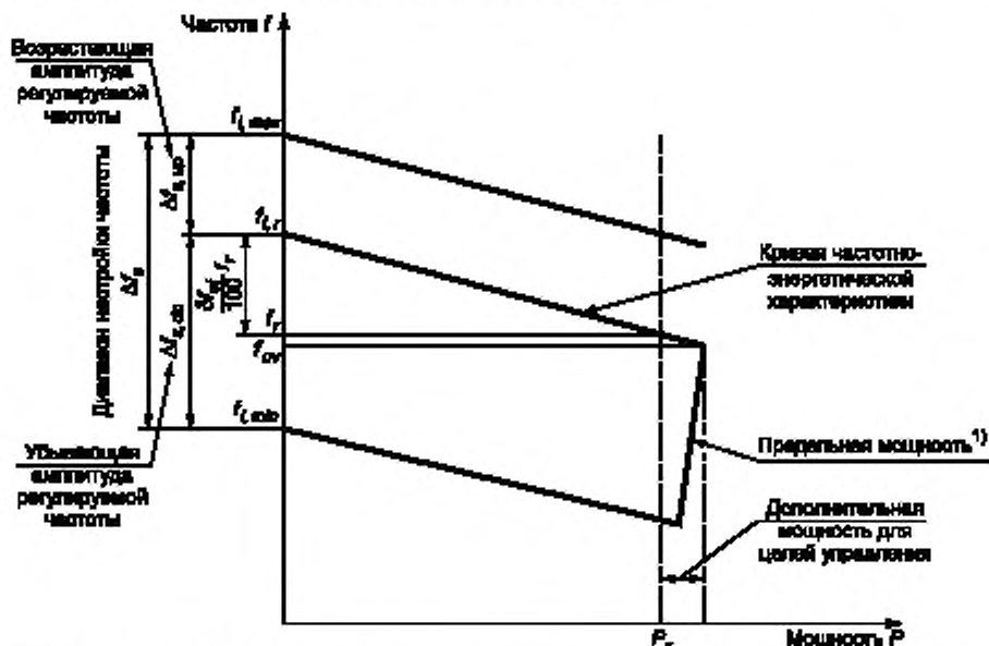
Рисунок 1 — Частотно-энергетическая характеристика диапазона регулируемой частоты
