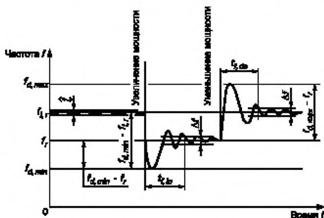
Рисунок 4 — Динамический режим частоты
