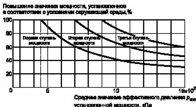
Рисунок 9 — Ориентировочные значения внезапных максимальных повышений мощности как функции тормозного эффективного среднего значения давления p_{\text{эф}} при объявленной мощности (двухтактные высокоскоростные двигатели)
