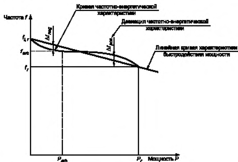
Рисунок 2 — Частотно-энергетическая характеристика отклонения от линейной кривой
