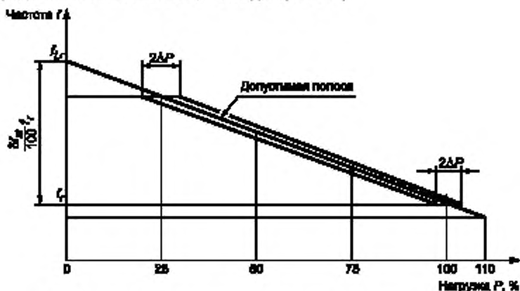
Рисунок 12 — Распределение мощности при параллельной нагрузке
