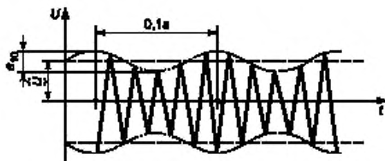
Рисунок 6 — Синусоидальная модуляция напряжения амплитудой U_m и регулярной частотой 10 Гц
