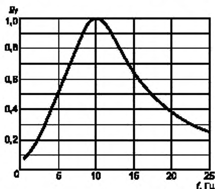
Рисунок 7 — Кривая эквивалентной восприимчивости в зависимости от изменения яркости
