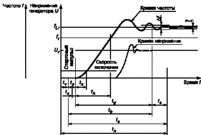
Рисунок 10 — Пусковые характеристики
