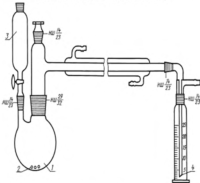
1 — колба перегонная; 2 — капилляры или пемза; 3 — воронка капельная; 4 — приемник
