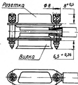
Черт. 24 Крепежный винт
