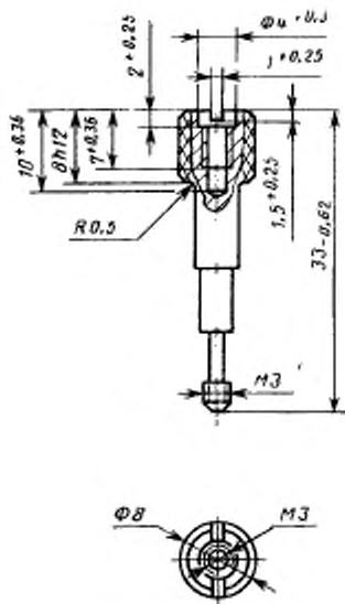
Черт. 24 Крепежный винт
