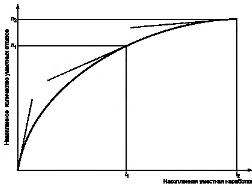
Рисунок 9 — Характерная кривая, показывающая мгновенные и экстраполируемые интенсивности отказов
