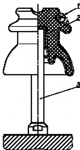
1 — провод; 2 — уплотнитель; 3 — штырь
