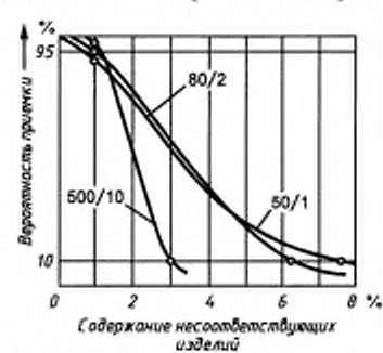
Кривые оперативных характеристик для планов выборочного контроля
