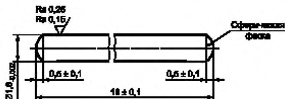
Рисунок 2 — Испытательный мандрен
