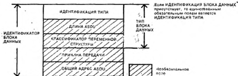
Рисунок 7 — Основная структура ИДЕНТИФИКАТОРА БЛОКА ДАННЫХ
