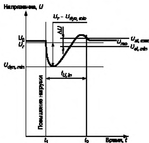
Рисунок А.1 — Характеристика переходного напряжения (повышение нагрузки)
