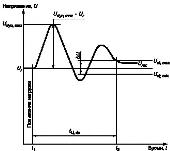
Рисунок А.2 — Характеристика переходного напряжения (понижение нагрузки)
