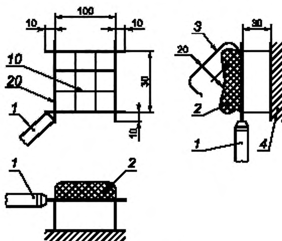
Рисунок А.1 — Рамка для закрепления ватного тампона
