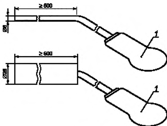
Рисунок А.2 — Конструкция щупов
