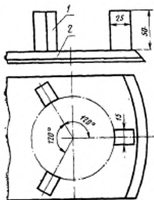
1—ограничитель; 2—подставка
