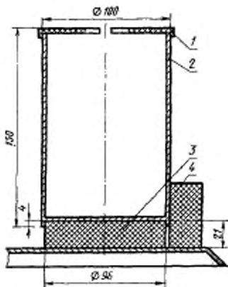
1—крышка; 2—стакан; 3—резиновая подставка; 4—ограничитель
