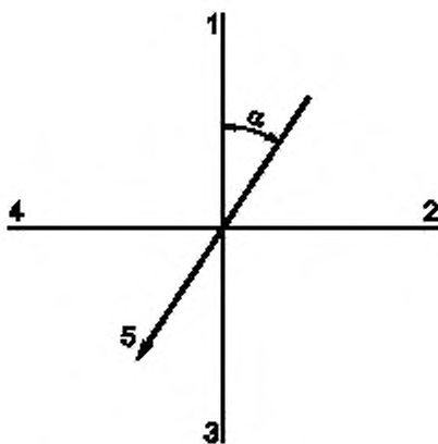
Рисунок В.1 — Угол направления ветра \alpha
