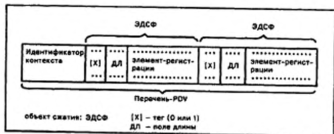
Рисунок 5 — Метод сжатия INTAR-СП1
