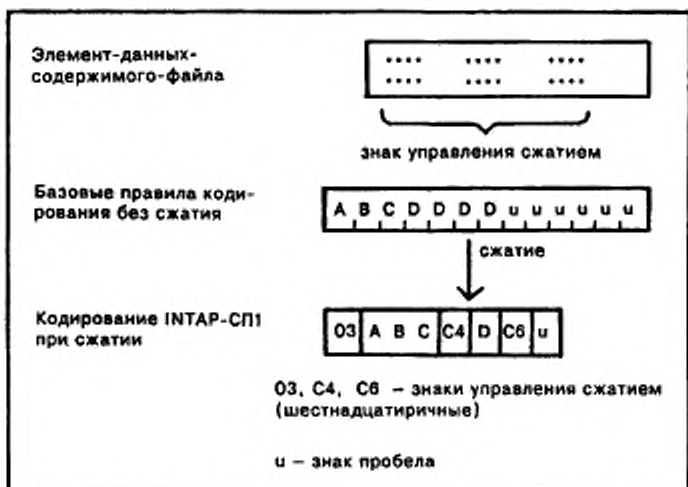
Рисунок 7 — Пример кодирования при использовании INTAR-СП1
