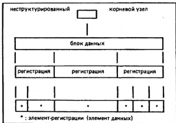
Рисунок 1 — Структура типа документа по INTAP—1
