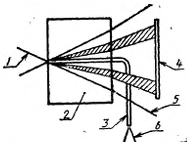
Метод преломления в ближнем поле. Схема
