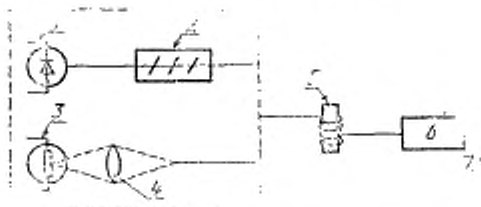
Аппаратура для измерения затухания на установленной длине волн
