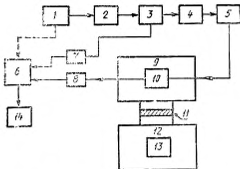
1 — модулированный источник света; 2 — оптические фильтры; монохроматор; 3 — оптический светодетектор; 4 — имитатор ввода на входе; 5 — устройство выделения мод оболочки; 6 — синхронный детектор; 7 — опорный детектор; 8 — оптический детектор; 9 — камера с регулируемой температурой; 10 — испытуемый образец; 11 — регистрирующее устройство; 12 — затвор; 13 — экранированная камера; 14 — источник гамма-излучения.
