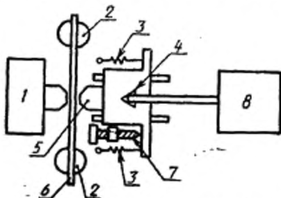
1 — неподвижный контакт; 2 — держатель образца; 3 — пружины; 4 — щуп; 5 — контакт на прецизионной платформе; 6 — образец; 7 — микрометрический винт; 8 — электронный микрометр
