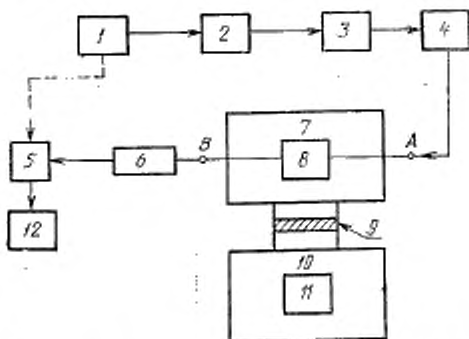
1 — модулированный источник света; 2 — оптические фильтры (монохроматор); 3 — имитатор ввода на входе; 4 — устройство выделения мод оболочки; 5 — синхронный детектор; 6 — оптический детектор; 7 — камера с регулируемой температурой; 8 — испытуемый образец; 9 — затвор; 10 — экранированная камера; 11 — источник гамма-излучения; 12 — регистрирующее устройство.
