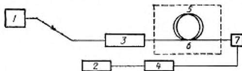
Схема установки для проведения испытаний с использованием стабилизированного источника
