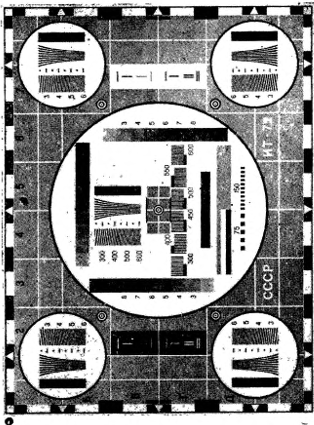
ВАРИАНТЫ ТЕЛЕВИЗИОННЫХ ИСПЫТАТЕЛЬНЫХ ТАБЛИЦ
