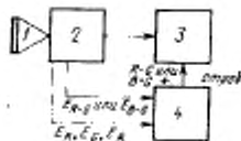
1 — испытательная таблица; 2 — камерный канал; 3 — ВКУ по п. 2.1.6; 4 — измеритель совмещения растров по п. 2.1.10
