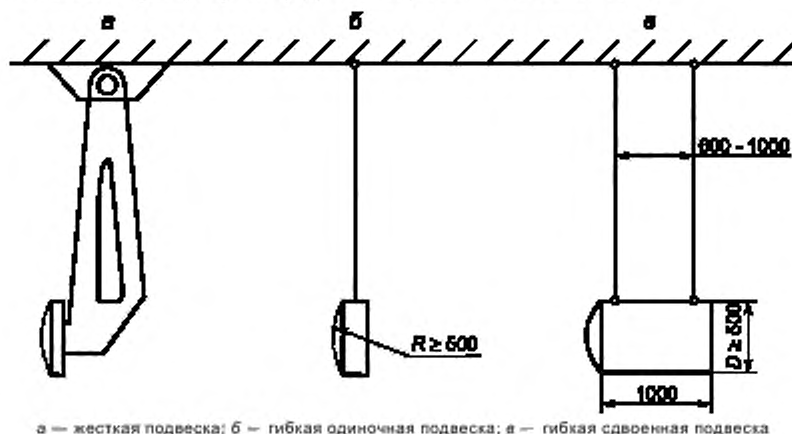
Рисунок 4 — Схема закрепления маятника
