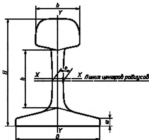
Рисунок 1 — Основные размеры поперечного сечения рельса
