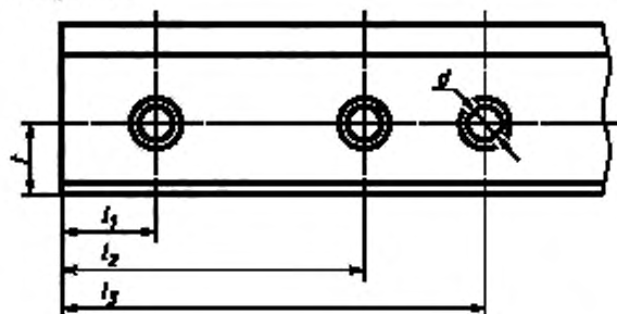
Рисунок 2 — Расположение болтовых отверстий
