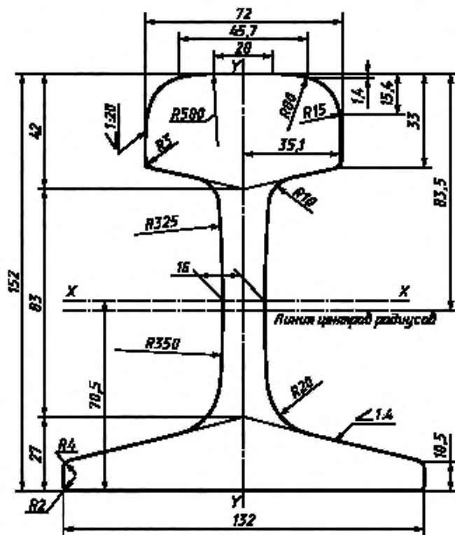
Рисунок А.1 — Рельс типа Р50
