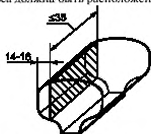
Рисунок 3 — Схема вырезки микрошлифа
