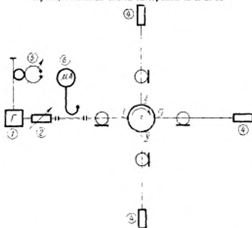
1—генератор; 2—аттенуатор; 3—испытываемый прибор; 4—нагрузка согласования; 5—резонатор; 6—микроамперметр
