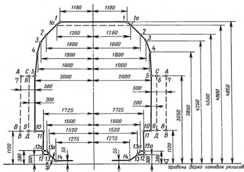
Габарит 1-СМ Верхнее очертание габарита
