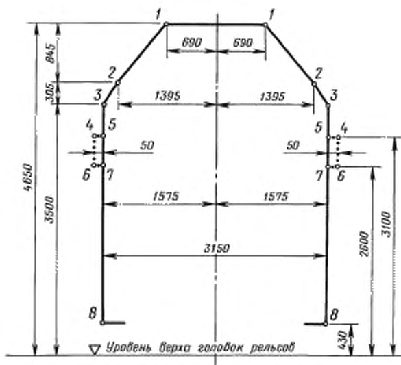
Габарит 02-ВМ Верхнее очертание габарита
