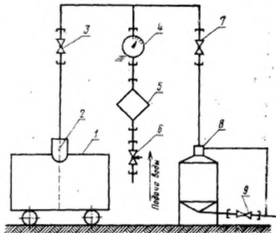
1—цистерна; 2—шланг; 3, 6, 7, 9—краны; 4—счетчик жидкости; 5—фильтр; 8—мерник
