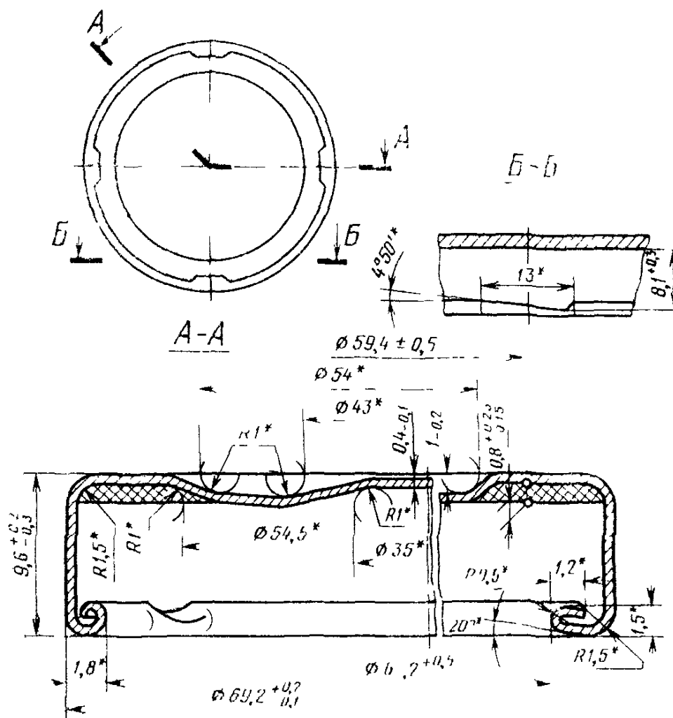
Размеры, обозначенные*, даны для изготовления инструмента Черт. 2
