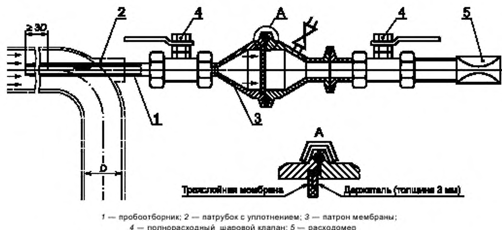
Рисунок 5 — Оборудование для изокинетического отбора проб в месте изгиба трубы по методу B2
