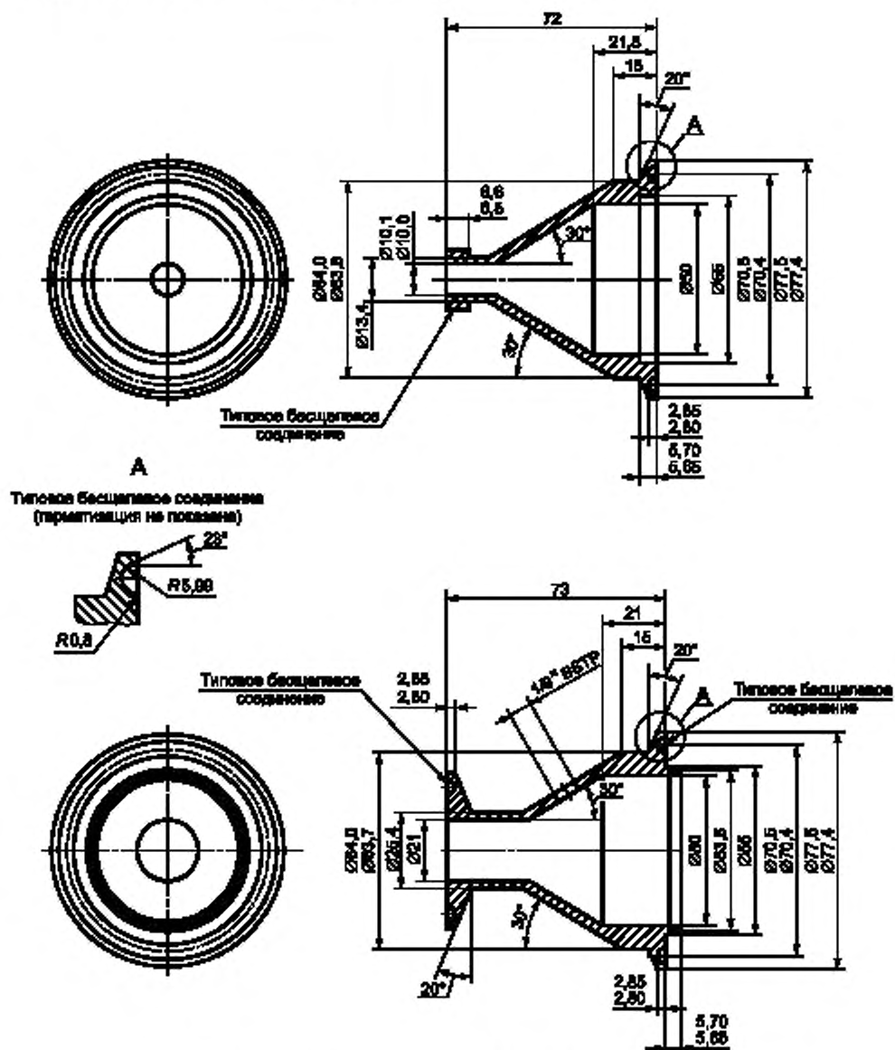
Рисунок 4 — Пример типового патрона мембраны
