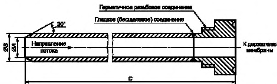
Рисунок 5 — Оборудование для изокинетического отбора проб в месте изгиба трубы по методу B2
