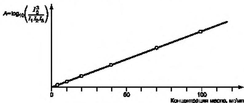
Рисунок 12 — Калибровочный график
