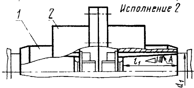
1 — втулка; 2 — обойма
