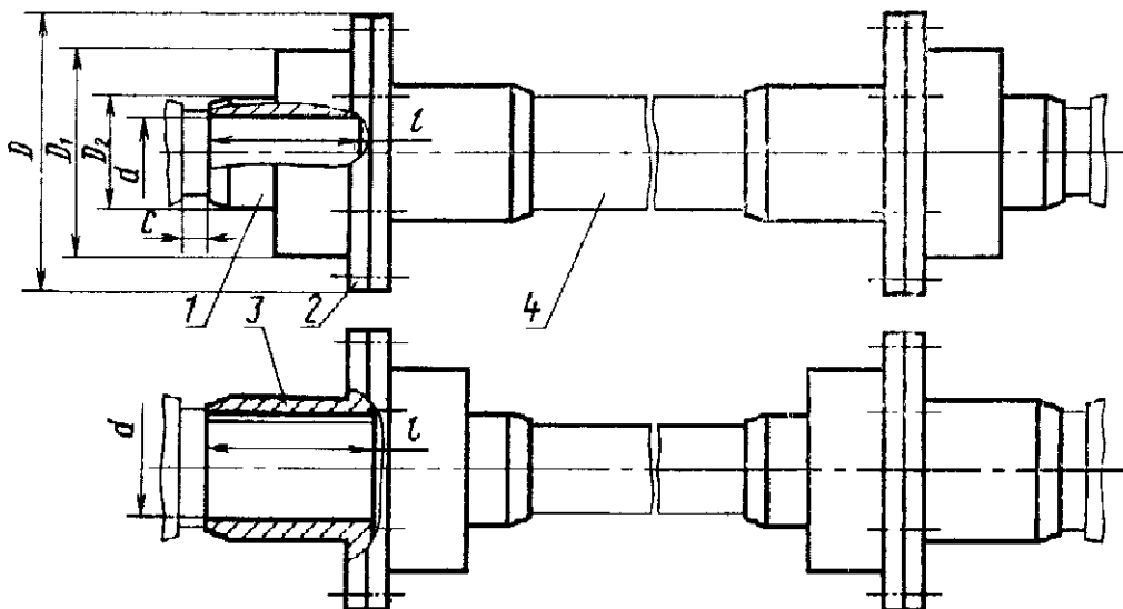
1—втулка; 2—обойма; 3—фланцевая полумуфта; 4—промежуточный вал
