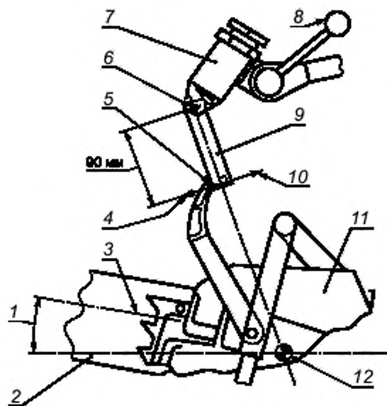
1 — угол выхода из образца; 2 — направляющая шина; 3 — центральная ось шины; 4 — направление измерения силы, приводящей в действие тормоз цепи; 5 — точка контакта; 6 — ось поворота; 7 — механизм регулировки рычага; 8 — положение рычага при испытаниях; 9 — подпружиненный рычаг; 10 — направление измерения силы отпуща рычага; 11 — силовой блок; 12 — центр тяжести
