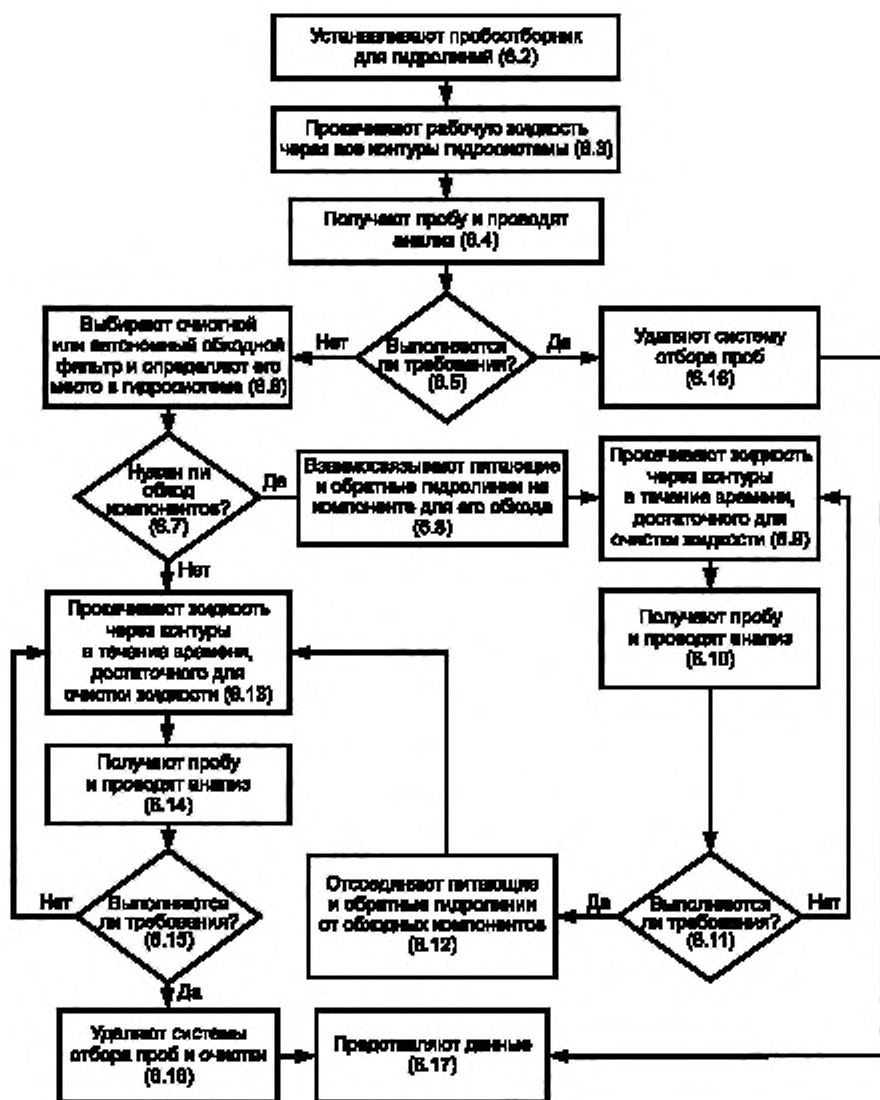
Рисунок 1 — Блок-схема, отражающая методику оценивания чистоты собранной гидросистемы
