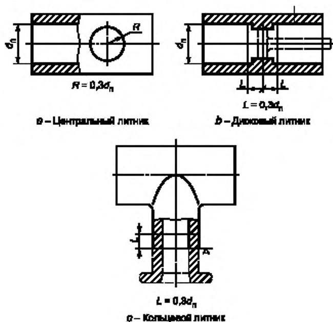
Рисунок 1 — Литниковые системы
