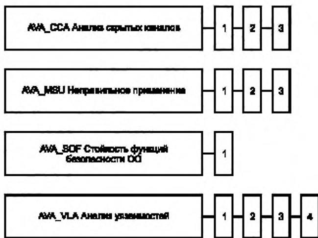
Рисунок 15 — Декомпозиция класса AVA: «Оценка уязвимостей»
