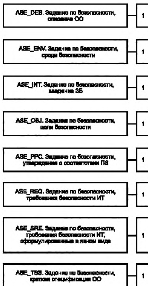
Рисунок 7 — Декомпозиция класса ASE «Оценка задания по безопасности»
