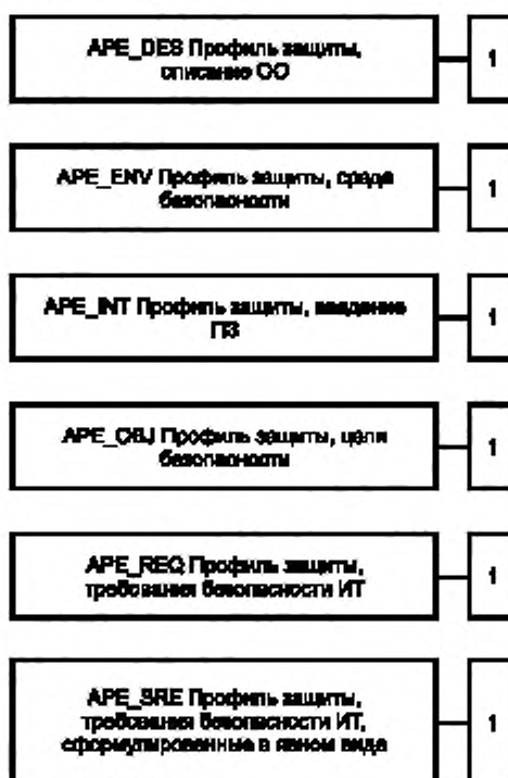
Рисунок 6 — Декомпозиция класса APE «Оценка профиля защиты»
