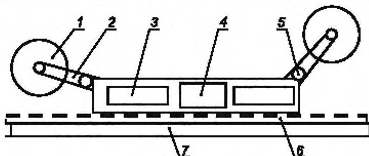
1 — шнек с резами; 2 — поворотный редуктор; 3 — отделение редуктора; 4 — взрывозащищенное распределительное устройство; 5 — взрывозащищенный шнековый электродвигатель; 6 — расположение ременной передачи; 7 — забойный скребковый конвейер
