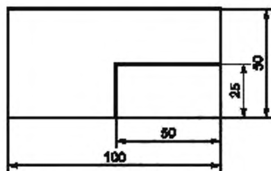
Рисунок 4 — Размеры образца для испытания
