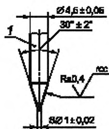
Рисунок 7 — Игла
