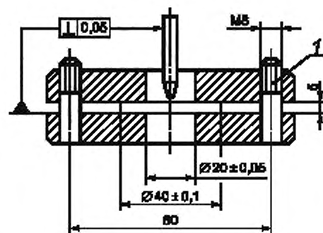
Рисунок 8 — Устройство для крепления образца
