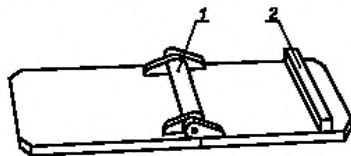
1 — стержень; 2 — упор
