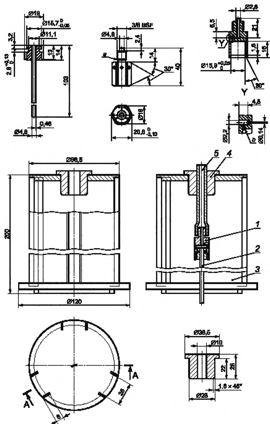
Рисунок 10 — Конструкция распылителя
