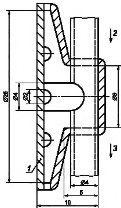
1 — ПВХ; 2 — осушающий воздух; 3 — проба, содержащая осушающий воздух
