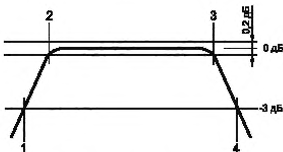
Рисунок В.1 — Характеристики полосового фильтра
