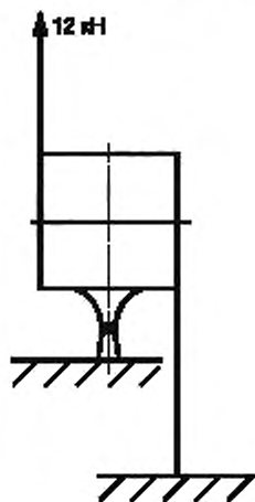
Рисунок 2 — Подвижное устройство
