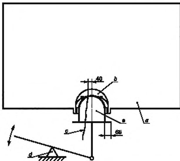
a — термокамера; b — образец для испытаний; c — термопара, d — подъемное устройство; e — термомакет головы
