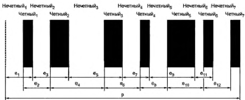
Рисунок 9 — Измеряемые параметры при декодировании
