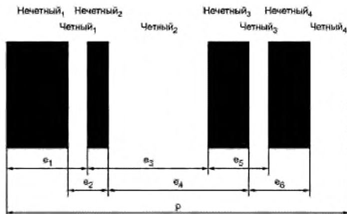
Рисунок 14 — Измеряемые параметры ширины при декодировании
