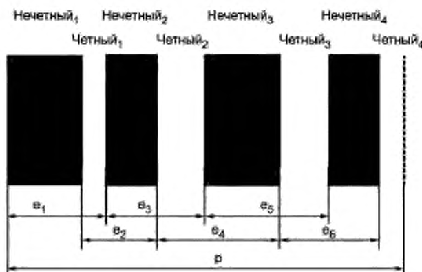
Рисунок 3 — Измеряемые размеры при декодировании
