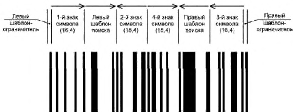
Рисунок 2 — Линейный символ GS1 DataBar Всенаправленный, представляющий номер (01)04412345678909
