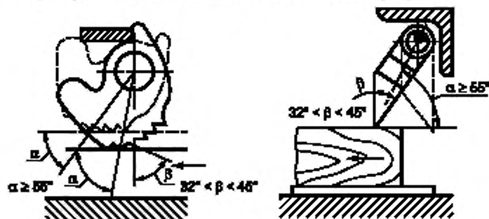
Рисунок 4 — качающиеся элементы (зубчатые секторы)
