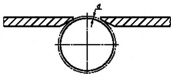
d — расстояние между кромками стола и диаметром окружности резания
