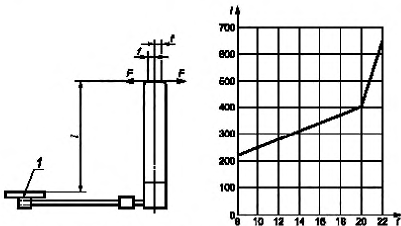
Рисунок А.1 — Наибольшая величина упругой деформации ограждения при испытании ограждения мостового типа
